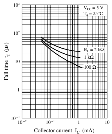
t_f - I_C
